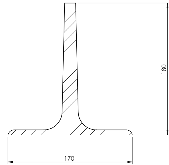
SEZIONE A-A
